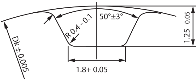
T5-Se
