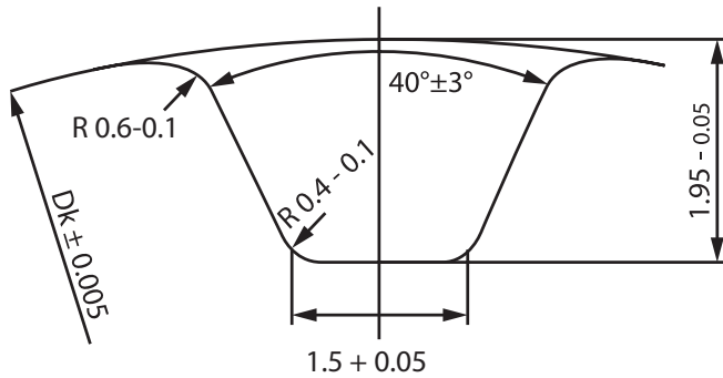
T5
