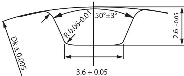
T10-Se
