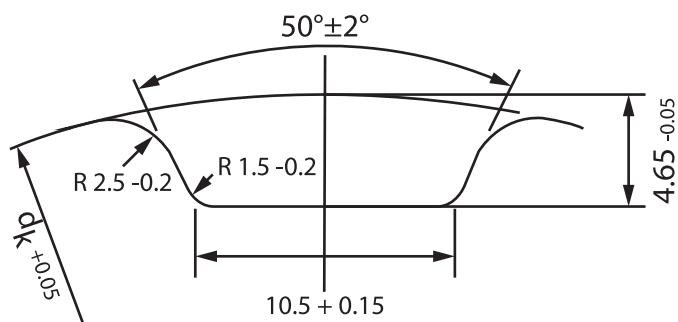
AT20
