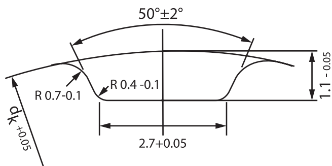
AT10A
